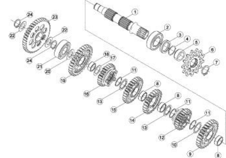
TAV.04B Albero secondario - Counter shaft - Arbre secondaire - Nebentriebwelle - Eje secundario
