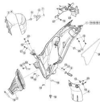
TAV.38 Scatola filtro - Filter box - Boî tier du filtre - Sicherungskasten - Caja del filtro
