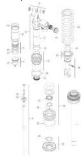
TAV.33A Ammortizzatore posteriore - Rear damper - Amortisseur arriere - Hinterer Stoßdämpfer - Amortiguador posterior
