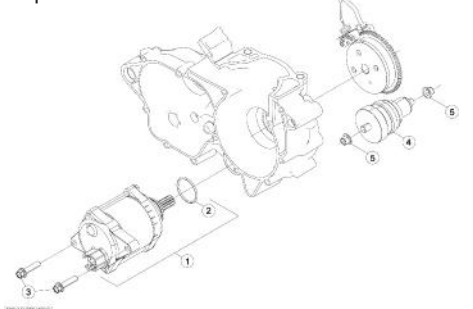
TAV.07 Avviamento elettrico - Electric starter - Dé marriage électrique - Elektrischer start - Arranque eléctrico
