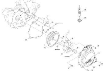
TAV.10 Gruppo accensione elettronica - Electronic ignition assy. - Groupe allumage électronique - Elektronischezündgruppe - Grupo encendido electrónico
