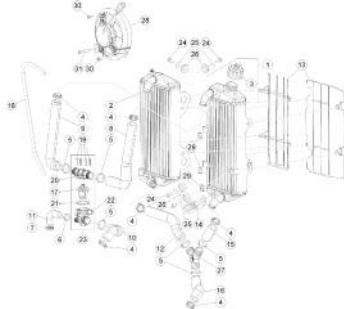
TAV.39 Impianto di raffreddamento - Installation de refroidissement - Installation de refroidissement - Kühlsystem - Instalaci3n de enfriamiento
