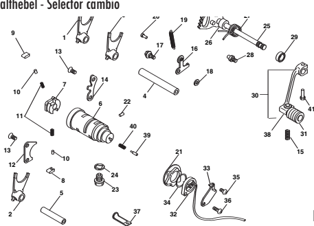
TAV.05 Selettore cambio - Gear selector - Selecteur changement de vitesses - Schalthebel - Selector cambio
