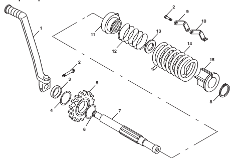
TAV.06 Avviamento a pedale - Starter pedal - Dé marrage à pedal - Kickstarter - Arranque a pedal
