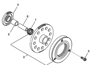
TAV.07B Avviamento elettrico - Electric starter - Dé marrage électrique - Elektronisch Anlassen - Arranque electrico
